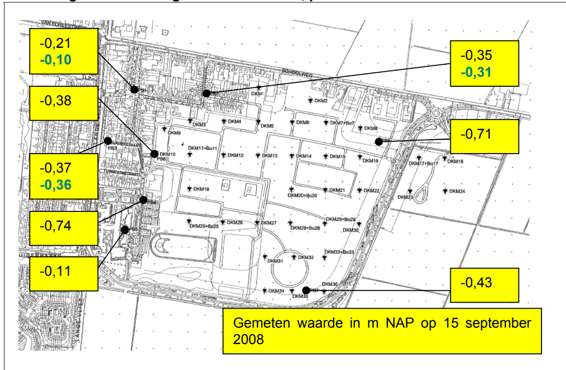
Afbeelding 2.1. Gemeten grondwaterstanden, peilbuizen 2008
