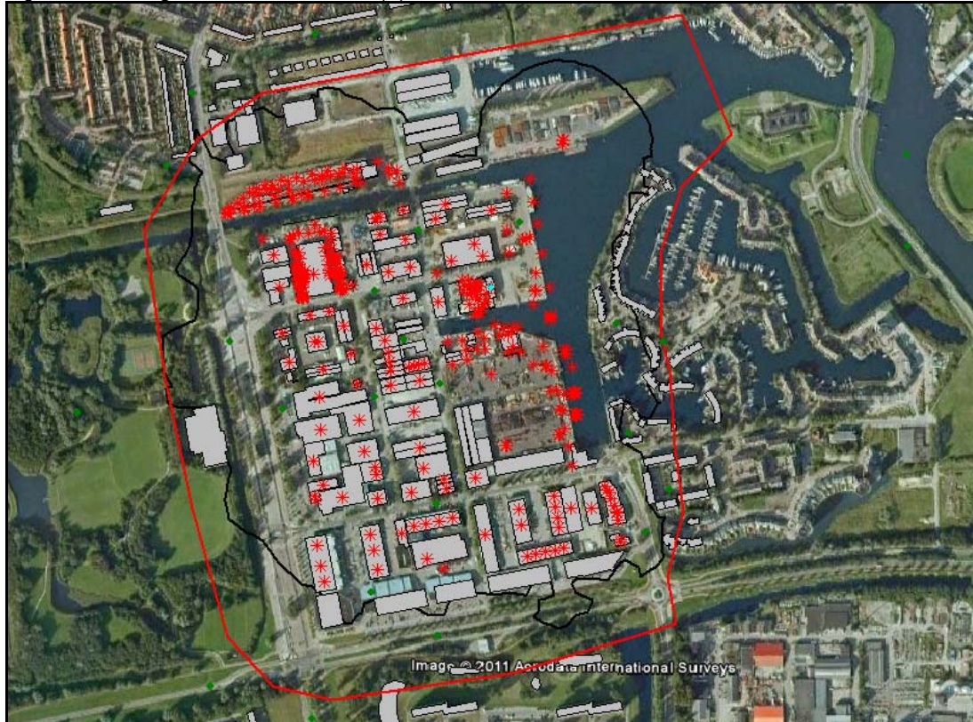
Figuur 5.1: zonegrens en actuele 50 dB(A) contour industrieterrein Westoever
