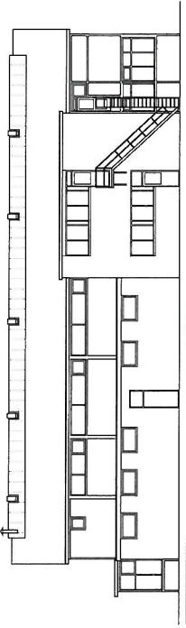
Zuidgevel
