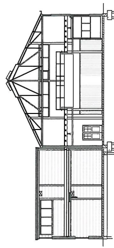
Doorsnede A-A
